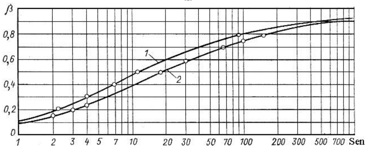
Рис. 1. Залежність коефіцієнту \beta від параметру Сен-Венана Sen : 1 – для труб \beta_T ; 2 – для кільцевого простору \beta_{кп}
